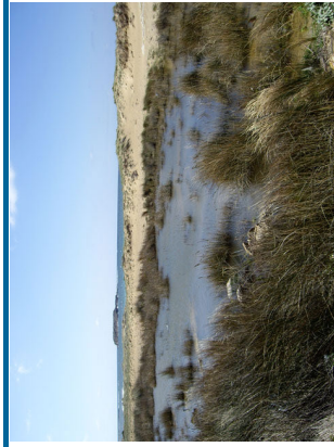
Εποχικό λιμνίο στα Φαλάκασαqρα
