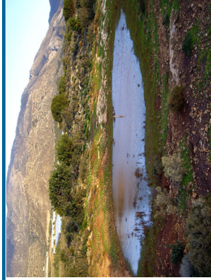
Οι ρουσιές στην περιοχή Χρυσοσκαλίτισσας-Ελαφονήσι
